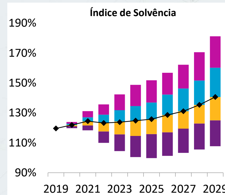
Carteiras que minimizem o risco de solvência no longo prazo
